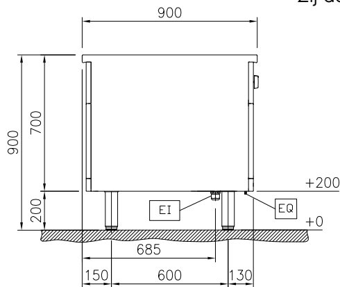
Zij aanzicht
